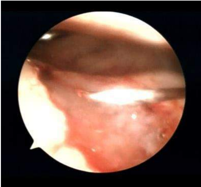
Iniezione Jointrep
